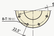
BGA-1,2,3,4のフランジ寸法
